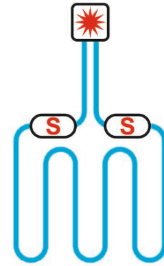
Схема укладки одножильного кабелю TXLP/1
